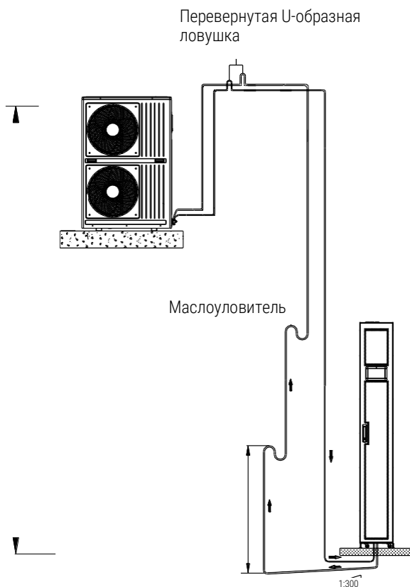
Рис. 3-1 Принципиальная схема установки положительного перепада
