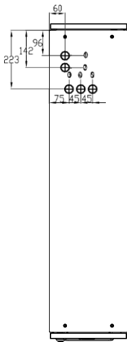
Верхняя часть
