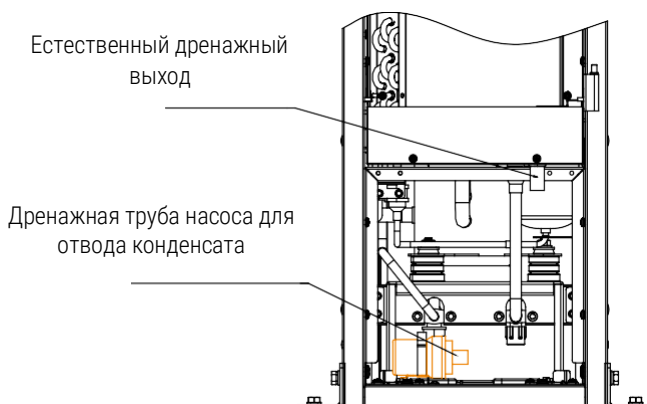
Рис. 3-8 Принципиальная схема положения стыка дренажных труб
