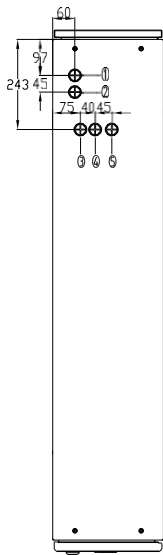
Верхняя часть
