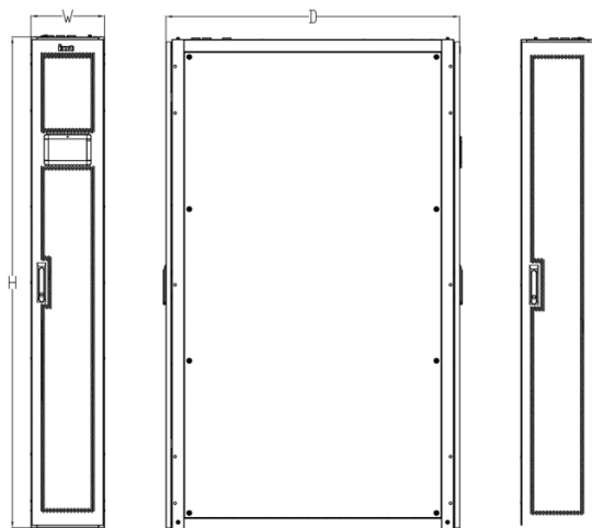
Спереди
