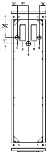
Опорная часть
