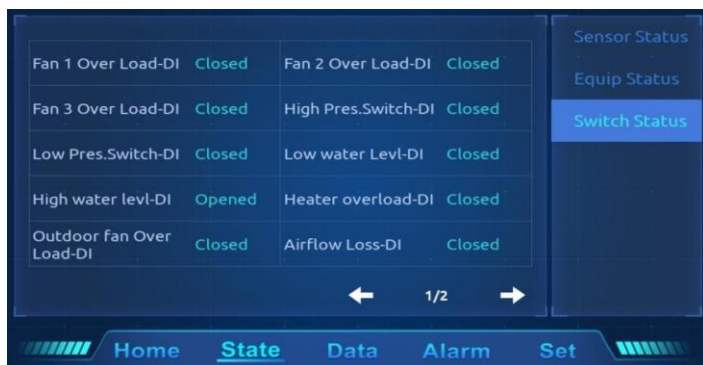
Рис. 4-5 Принципиальная схема состояния переключателя
